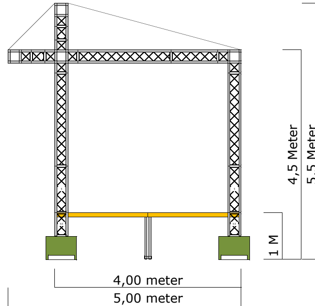
Zij aanzicht
