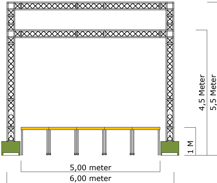
Voor aanzicht
