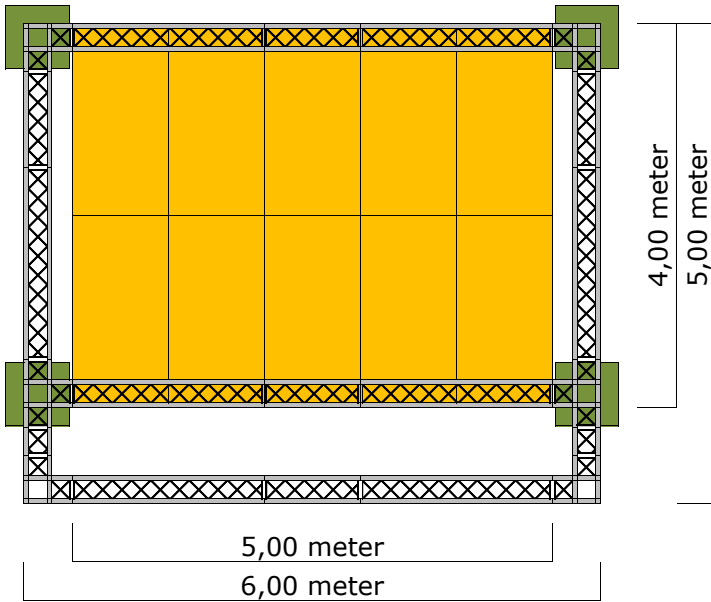
Boven aanzicht
