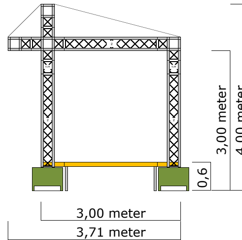
Zij aanzicht
