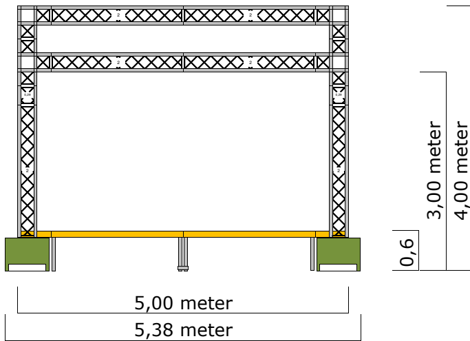
Voor aanzicht
