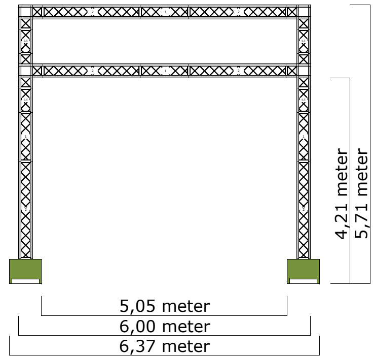
Zij aanzicht
