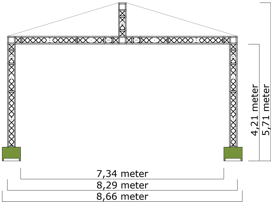
Voor aanzicht
