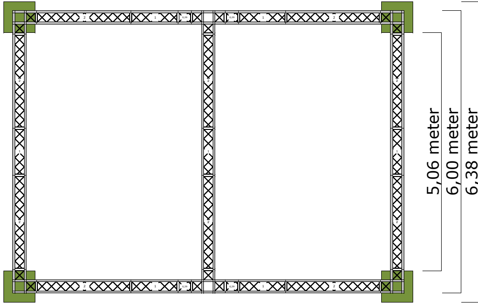
Boven aanzicht
